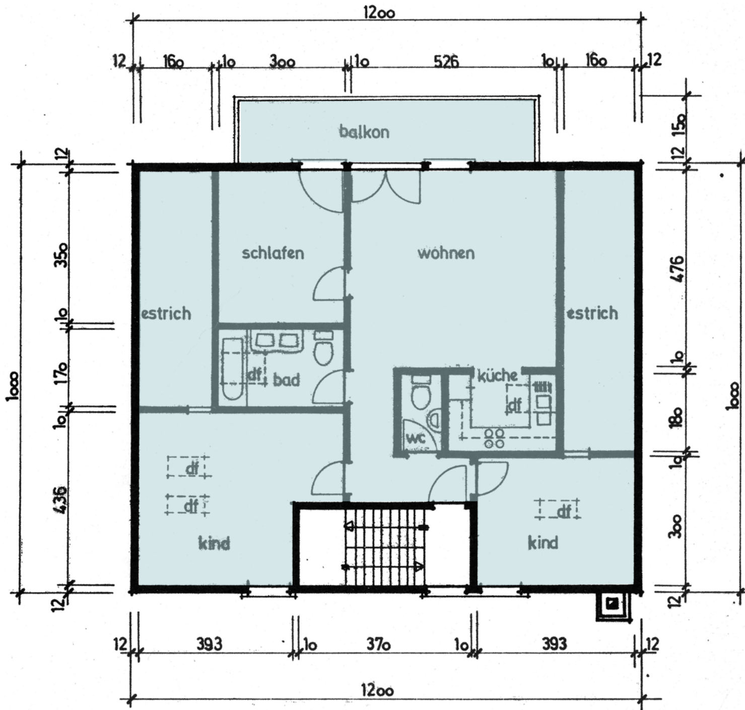
HÜTTETÜRLISTRASSE 17, 3718 KANDERSTEG 4 Zimmer Attikawohnung Grundriss
